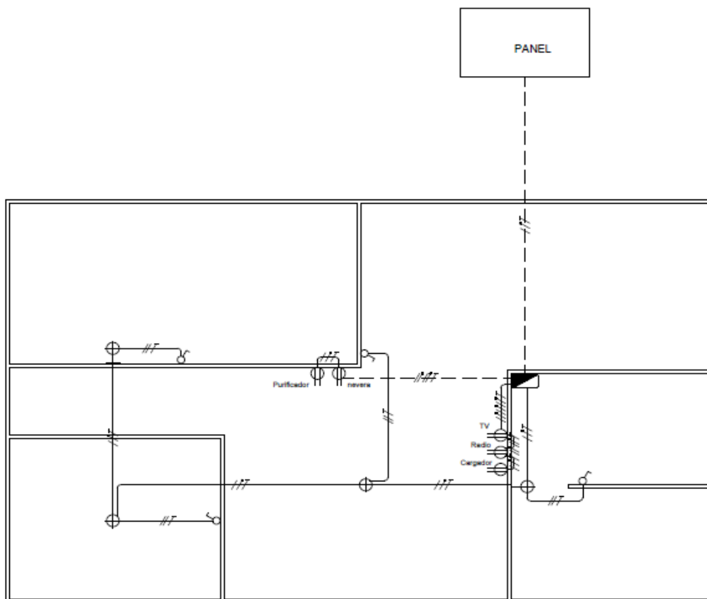
Ilustración 2 Instalaciones eléctricas internas (ejemplo)
